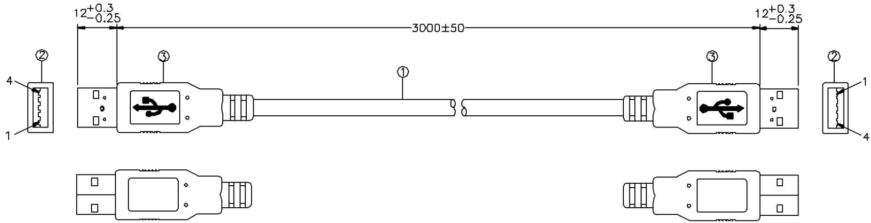
Conn.1 USB A Male Molding
